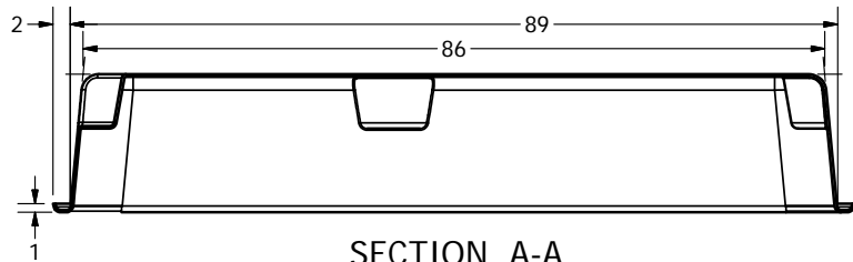
SECTION A-A SCALE 1:16
